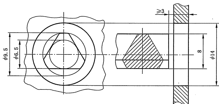
图 B.1 开锁三角形钥匙
