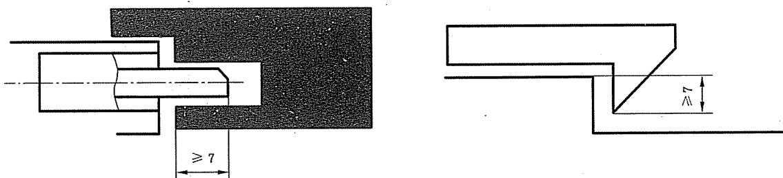
图 3 锁紧元件示例
