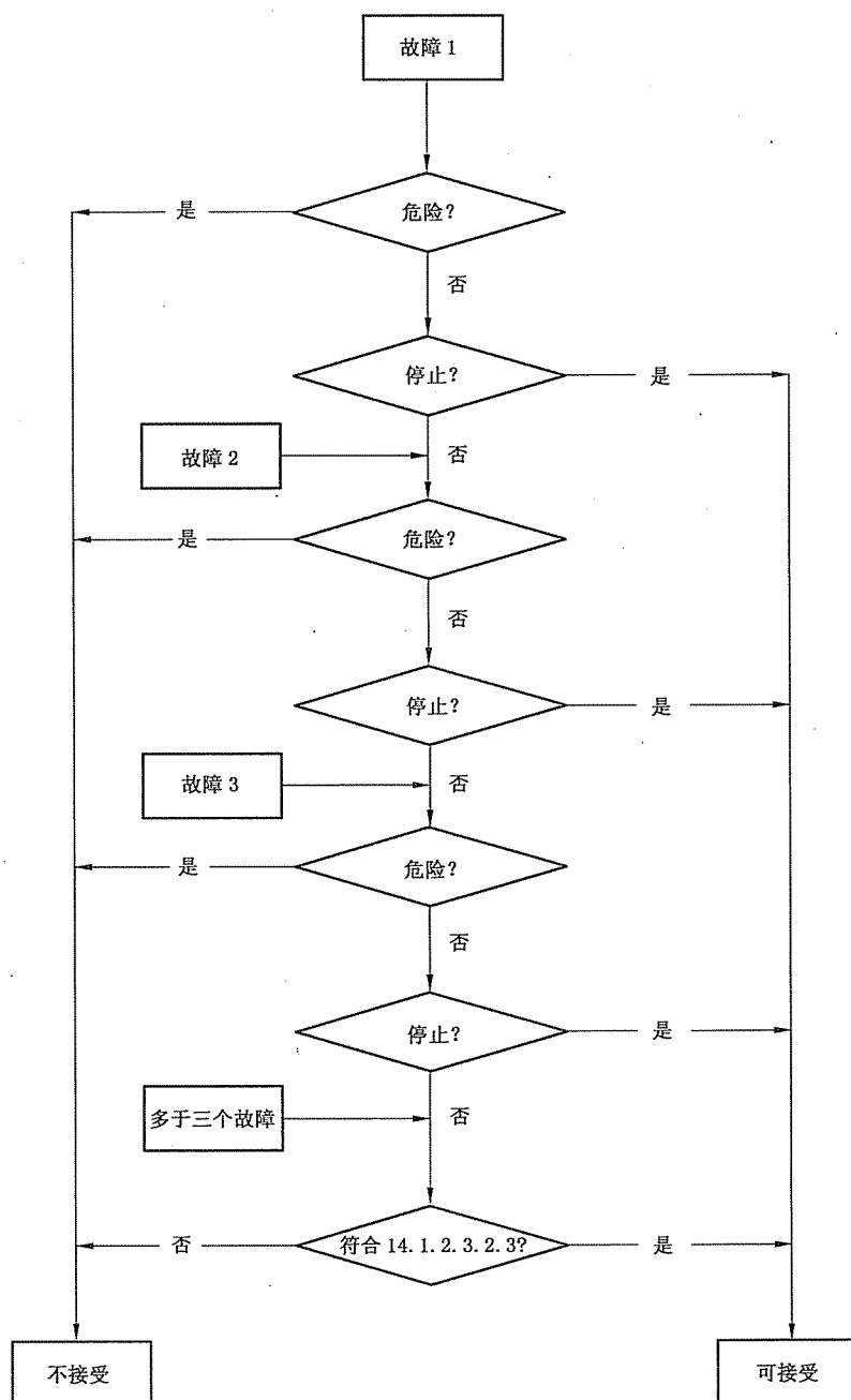
图6 安全电路评价流程图
