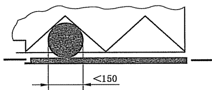
图 5 铰链层门和折叠轿门的间隙
