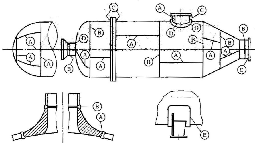
图 1 焊接接头分类
